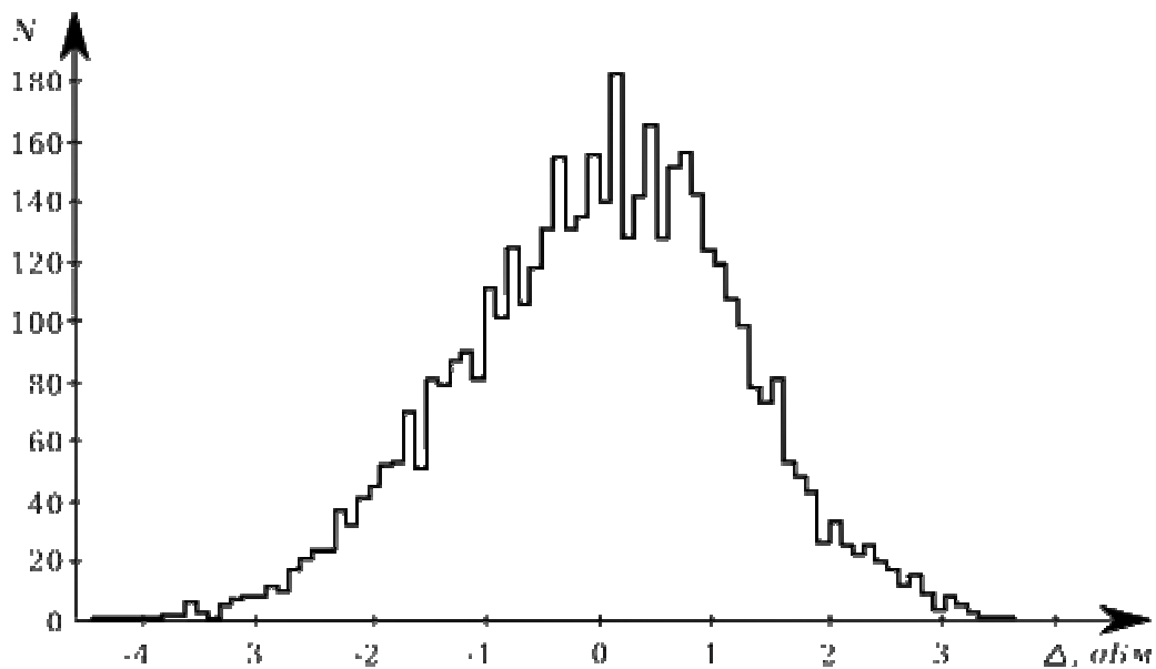
На рис. 1. Гистограмма абсолютных ошибок измерений.
